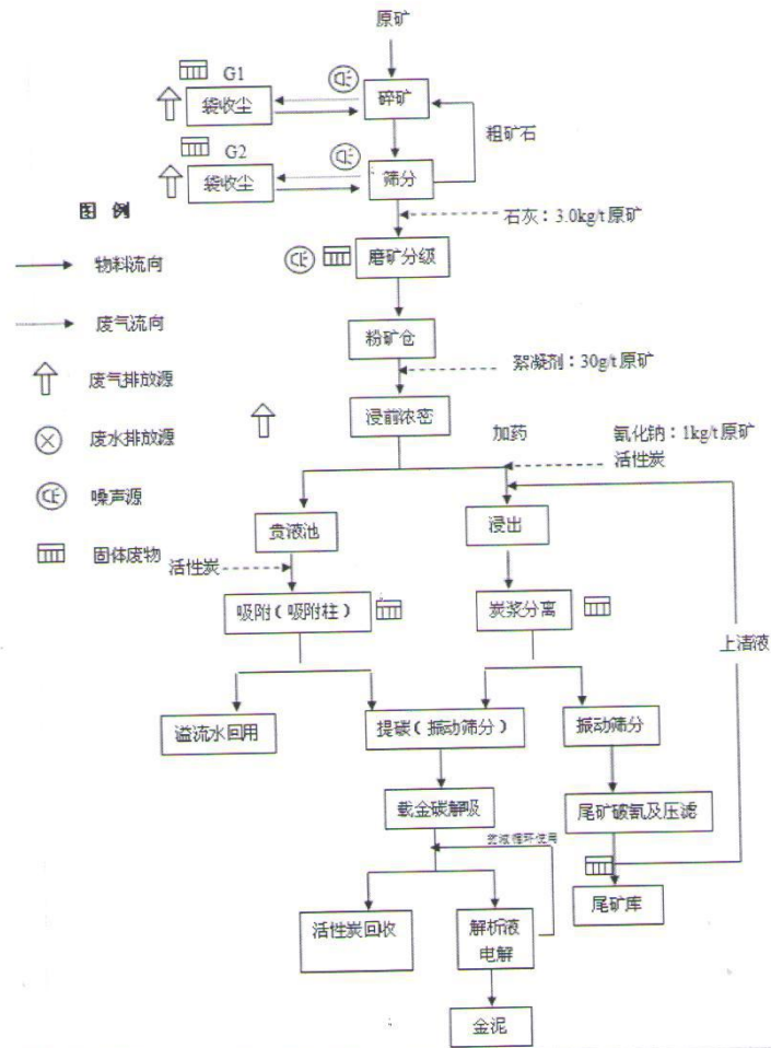
生产工艺流程图：
