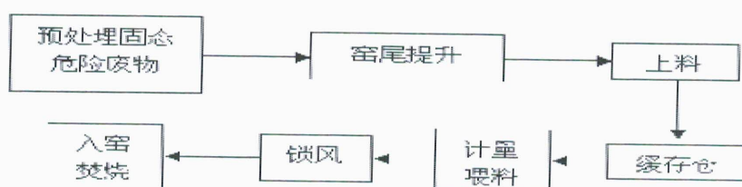
固态危险废物处置工艺流程
