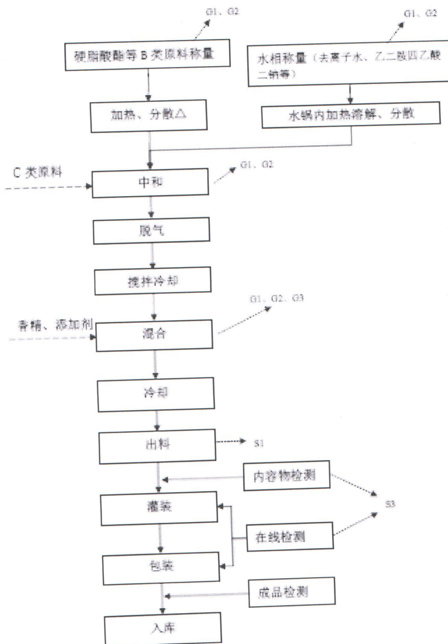
图 4.1-1 护肤类清洁产品生产工艺流程图
