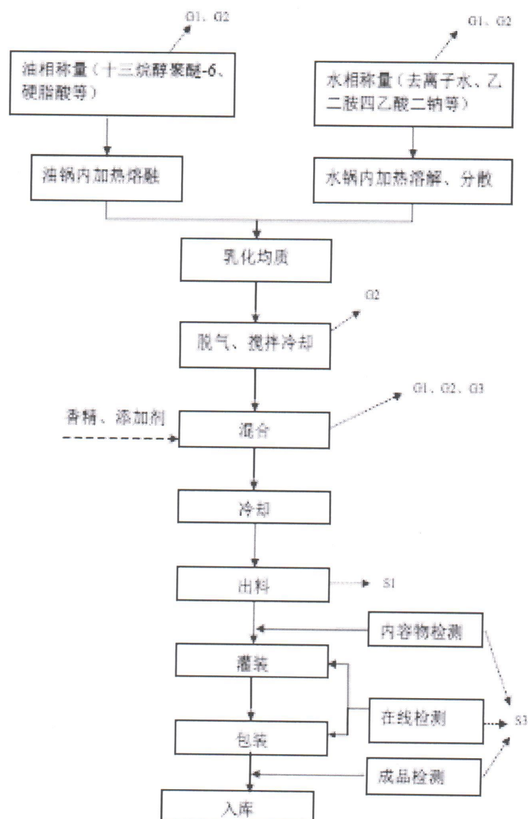
图 4.1-5 BB 霜产品生产工艺流程图
