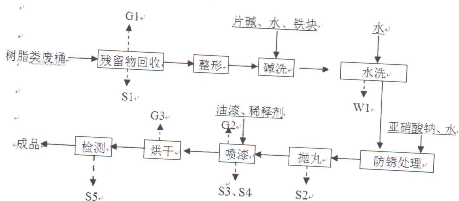
树脂类废桶回收工艺流程图
