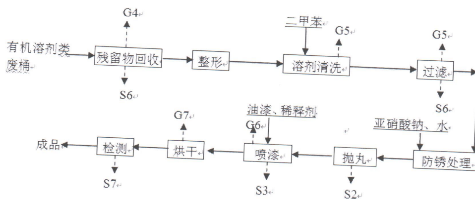
有机溶剂类废桶回收工艺流程图
