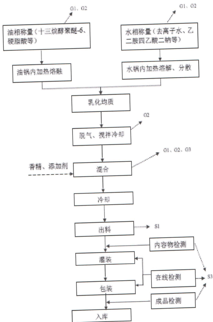
图 4.1-5 BB 霜产品生产工艺流程图
