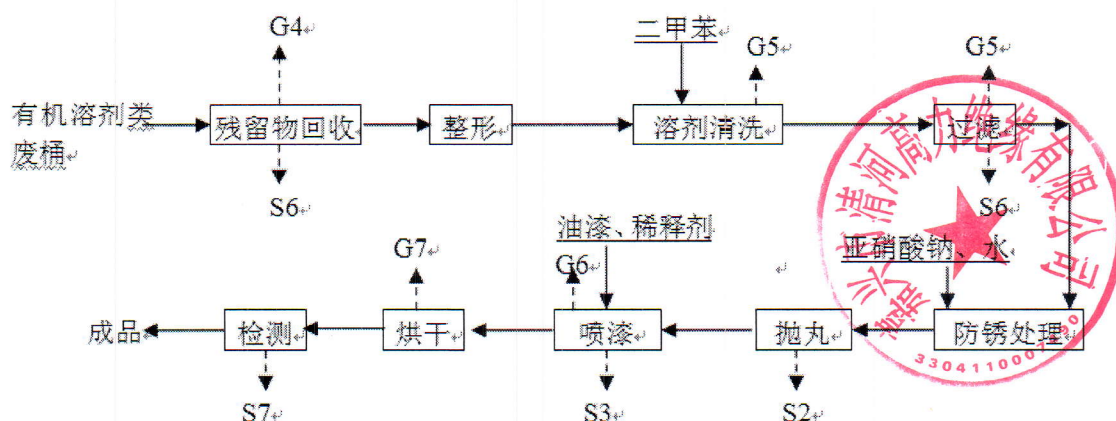
有机溶剂类废桶回收工艺流程图
